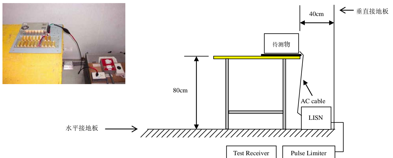
图一: 明纬 EMI 测试系统配置图
